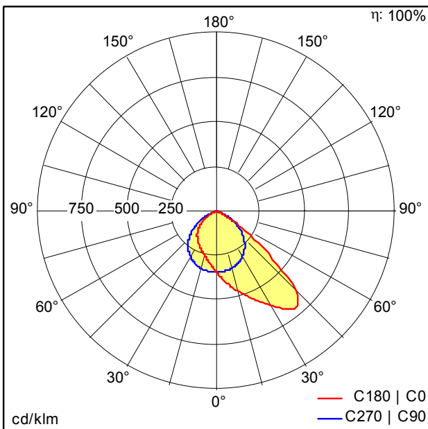
TE_LEO_FLEX_120W_830_FLEX1.idt
